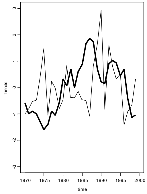
DFA2 and PPCA2
